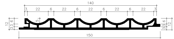
M150Y 内圆板
