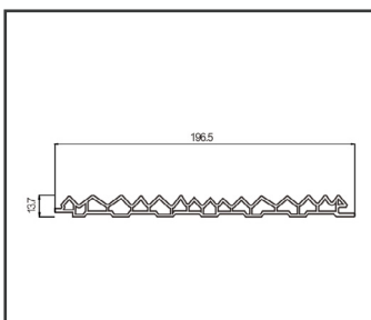
Item:M190 三角板
