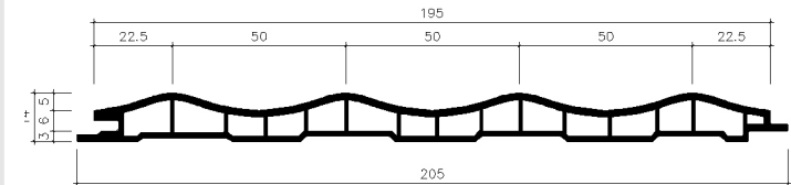
M205 外圆板
