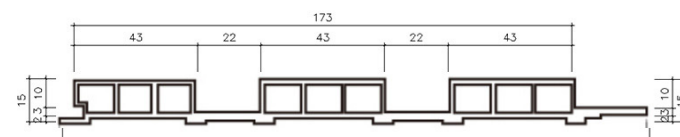
M204 长城板
