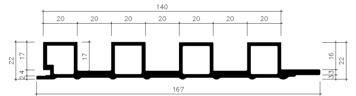
M170 格栅
