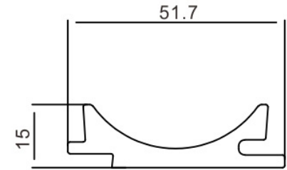
S50 半月板
