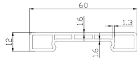
P60 (平线)
