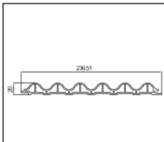
Item:M240 圆弧板
