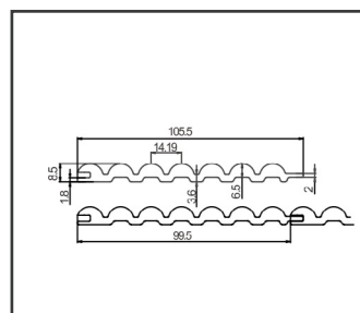
Item:S105 小圆板
