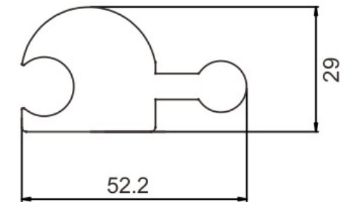
SH52Y 圆弧
