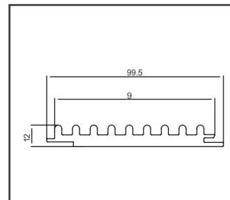
Item:SM100 波浪板
