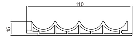
MT110 内圆板
