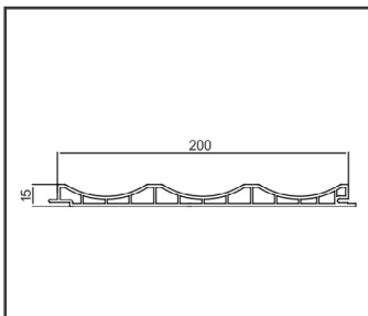
Item:M210 三圆板
