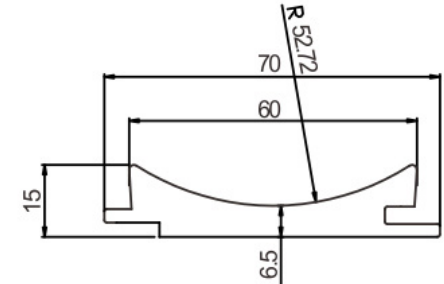
S7015 半月板
