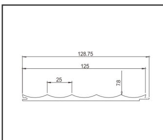
Item:S125 波浪板
