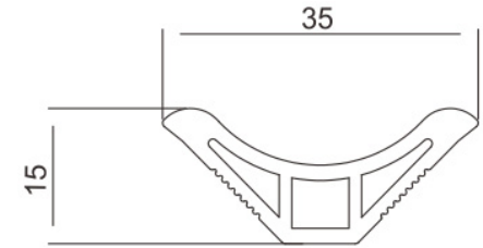
Y35 阴角线
