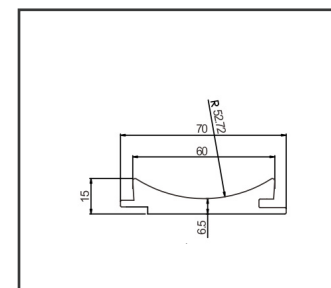
Item:S7015 半月板
