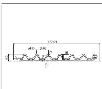
Item:M178 内圆板
